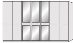
7 Door Robe 350cm(W) x 58cm(D) x 220cm (H)
